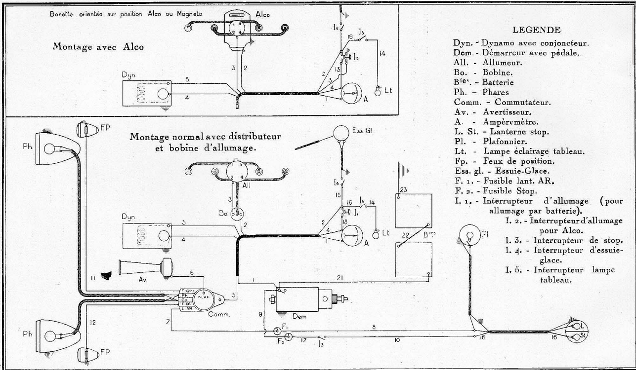
Fig. 27. — Schéma de l'installation électrique.
