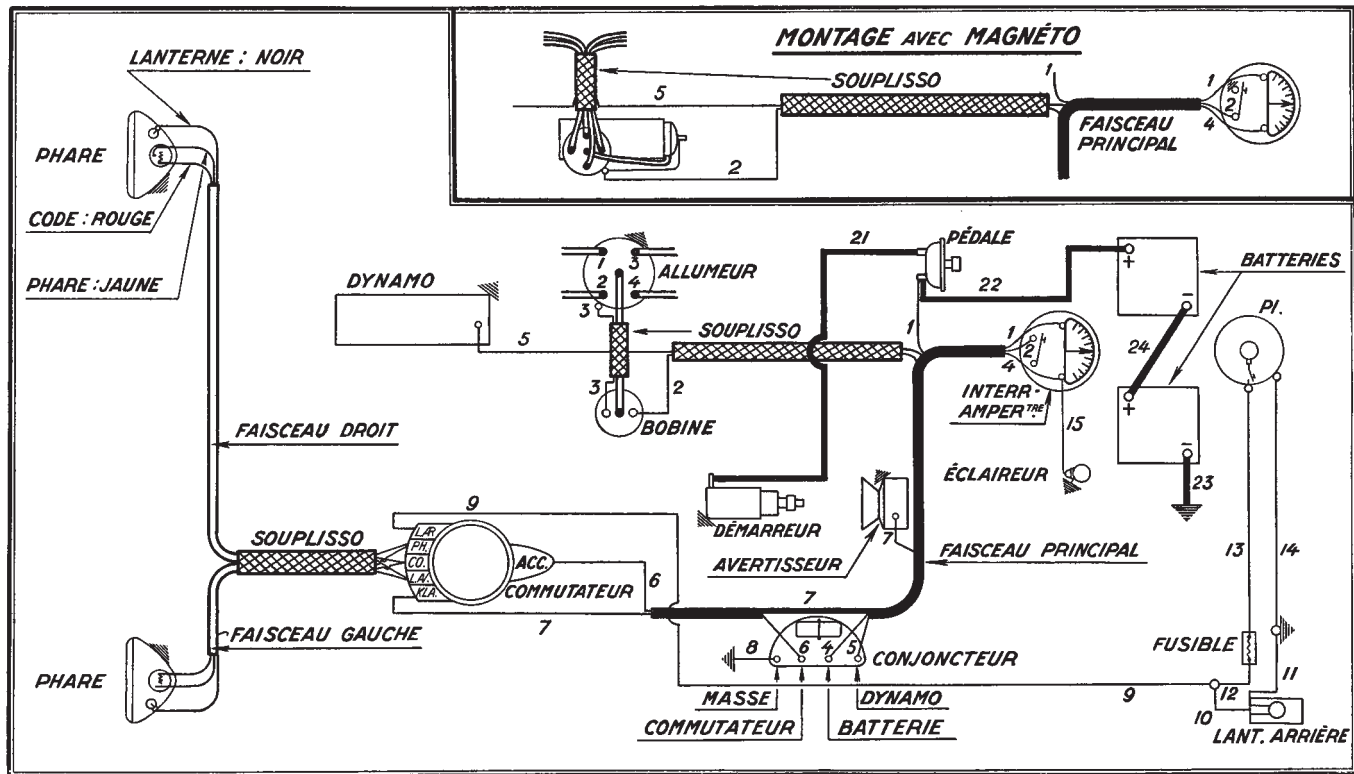
Fig. 25. — Schéma de l'installation électrique.
